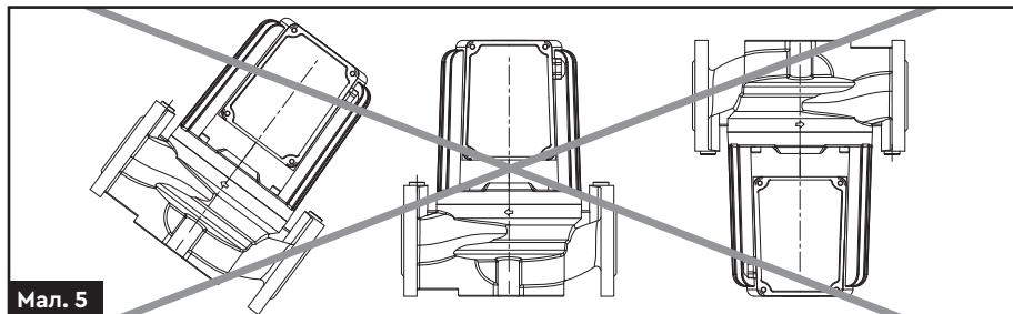
Мал. 5 – Помилки монтажу насоса
