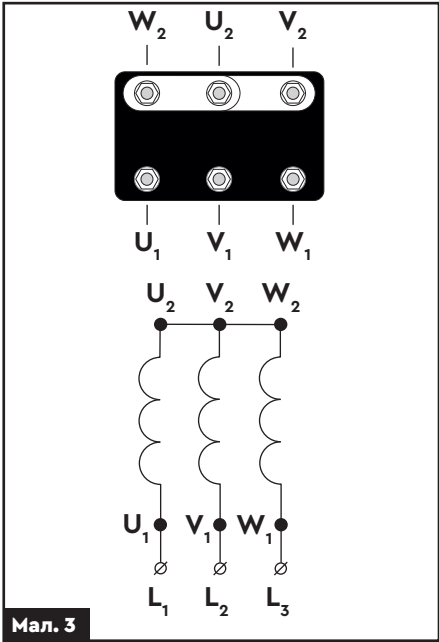
Схема «зірка» (мал. 3)
