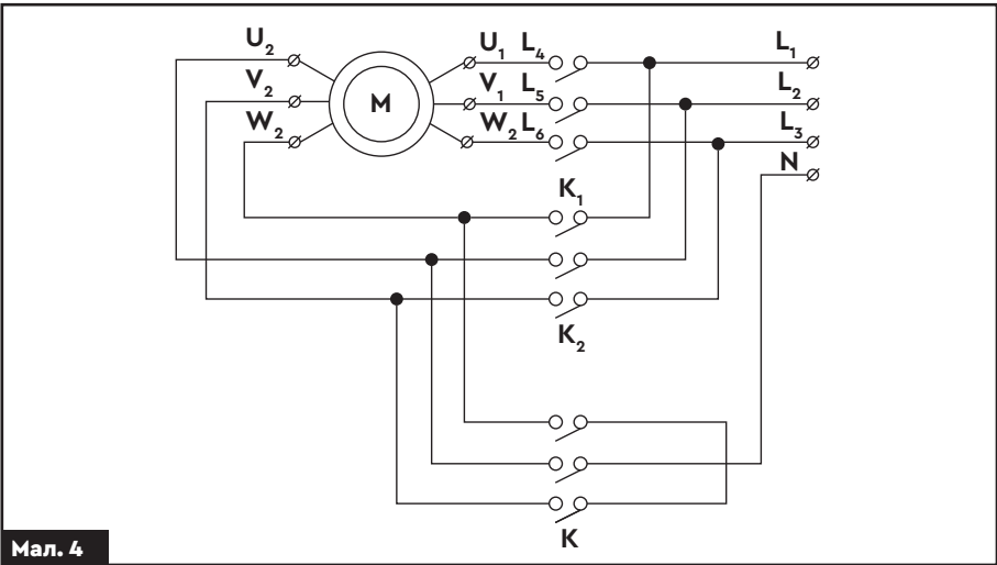
Комбінована схема «зірка-трикутник» (мал.4)
