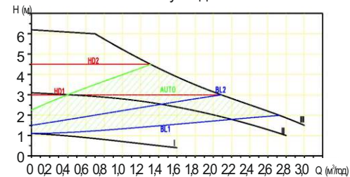
Діаграма характеристик насосу моделі 774136
