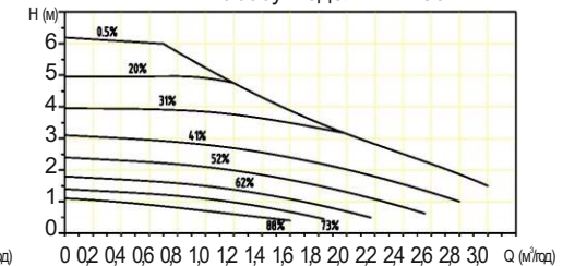
Діаграма характеристик по сигнальному управлінню PWM насосу моделі 774136
