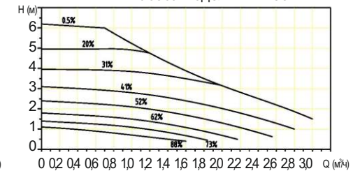
Диаграмма характеристик по сигнальному управлению PWM насоса модели 774136
