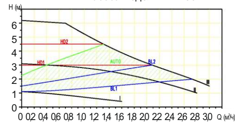
Диаграмма характеристик насоса модели 774136
