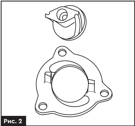
Рис. 2 – Деталі ріжучого механізму
